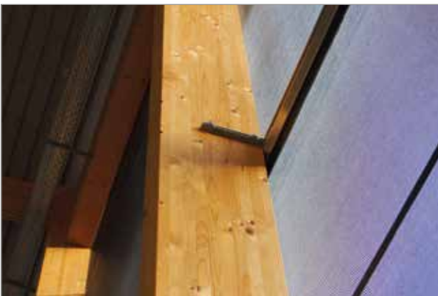
Detailansicht Befestigung
