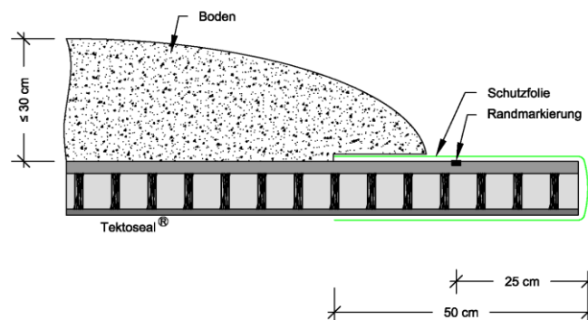
Abb 3. Temporäre Randsicherung
