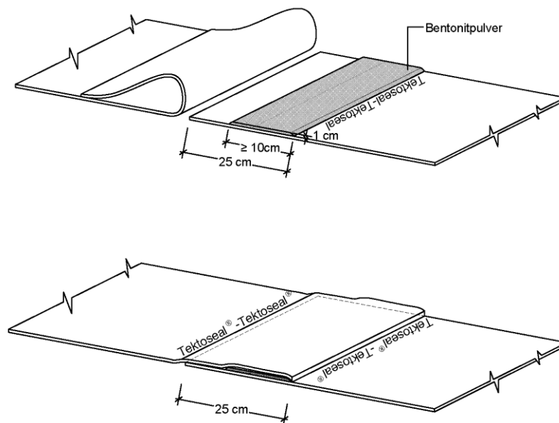
Abb. 6: Ausführung der Überlappung mit Bentonitpulver bzw. -paste
