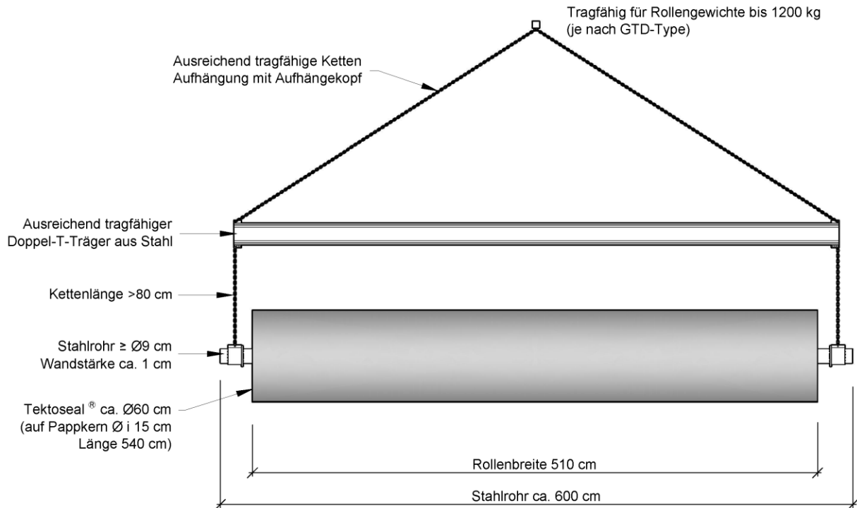
Abb. 1: Hebetraverse
