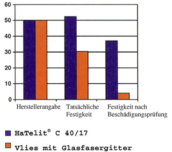
Diagramm 1. Ergebnisse der Zugkraftprüfungen
